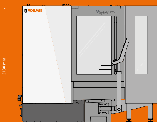
////// DIMENSIONES DE LA MÁQUINA VHybrid 260 con HC 4
